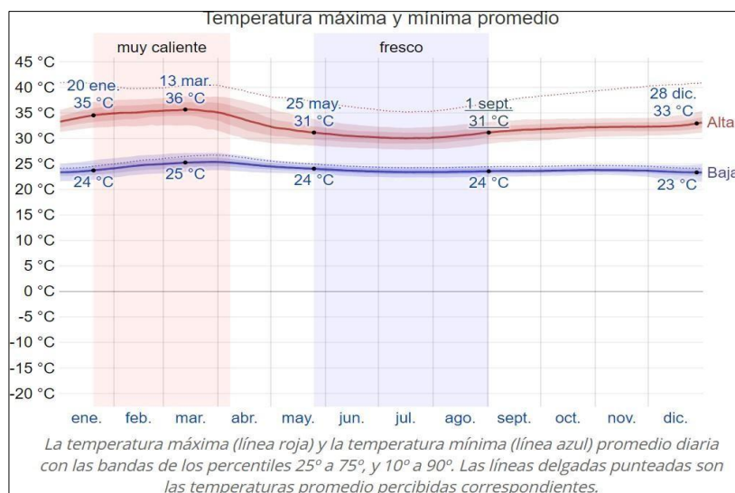
Temperatura máxima y mínima promedio de Puerto Carreño.
