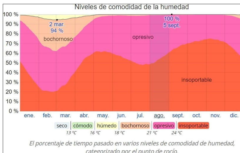
Niveles de comodidad de la Humedad.
